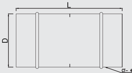
CT1 : CHI TIẾT CẢNH VAN/ DETAIL STRUCTURE WING
