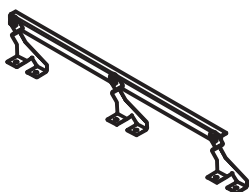
CT5 : LIÊN KẾT CÁNH VAN/ SHAFT TOGETHER CONNECT WING TÔN MẠ KẼM DÀY-1.15MM/ GALVANISED T-1.15MM
